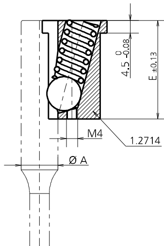
INSERT DIMENSIONS
